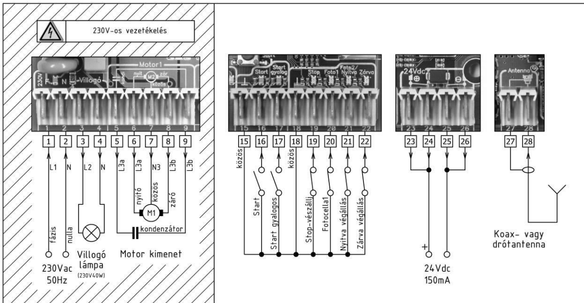
Sorcsatlakozók bekötése
